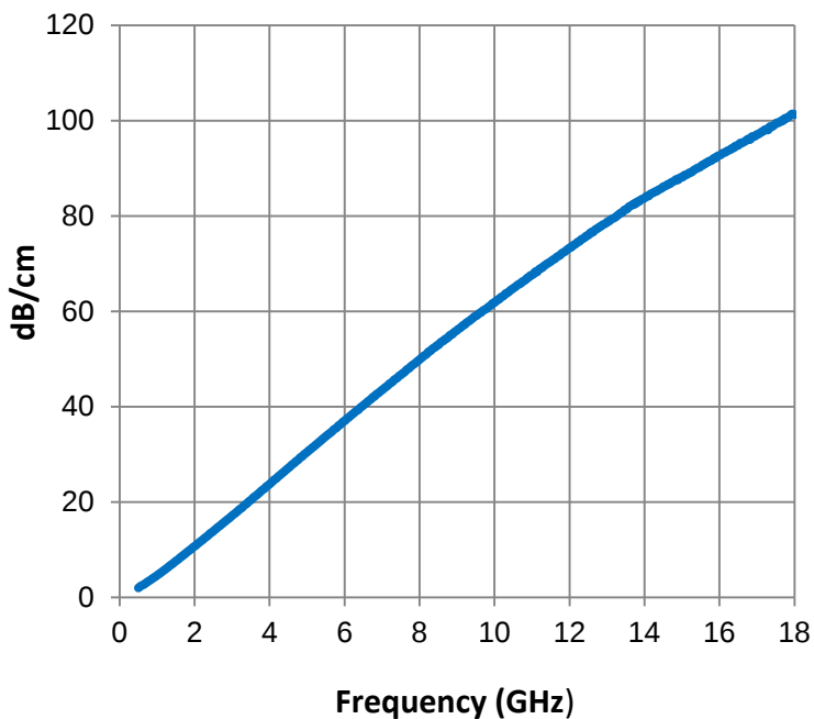
Attenuation
