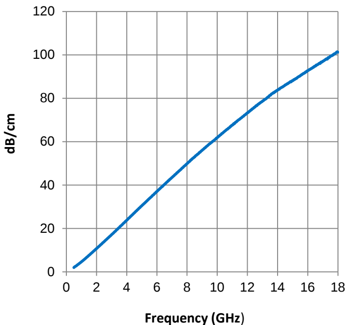
Attenuation
