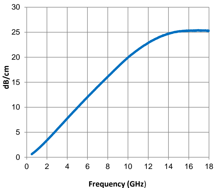
Attenuation
