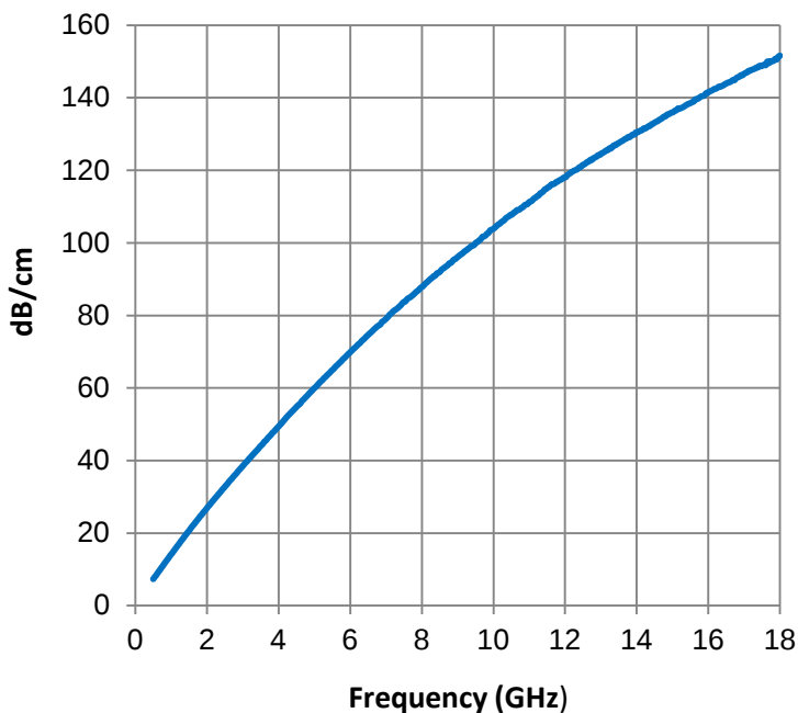
Attenuation
