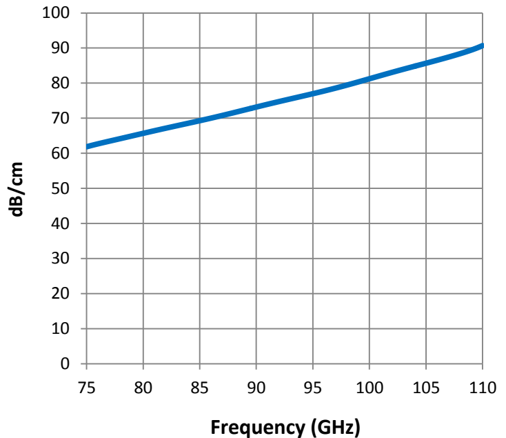
Attenuation
