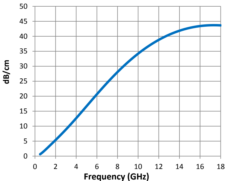
Attenuation
