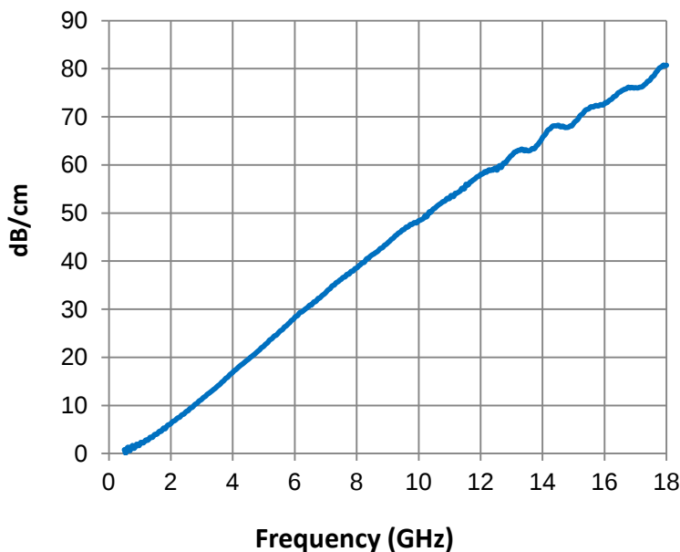
Attenuation
