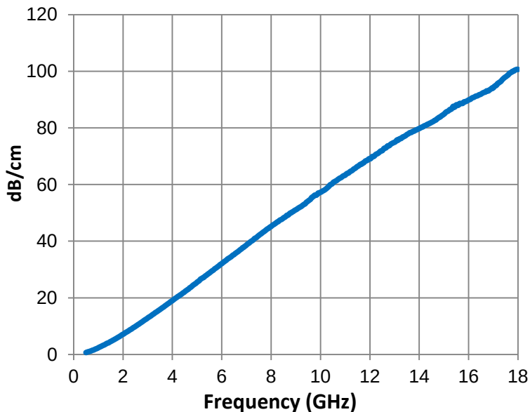
Attenuation
