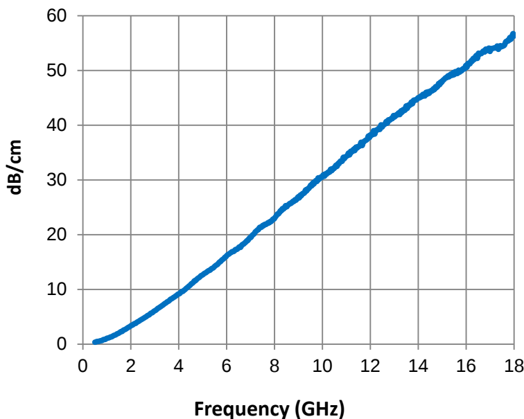
Attenuation
