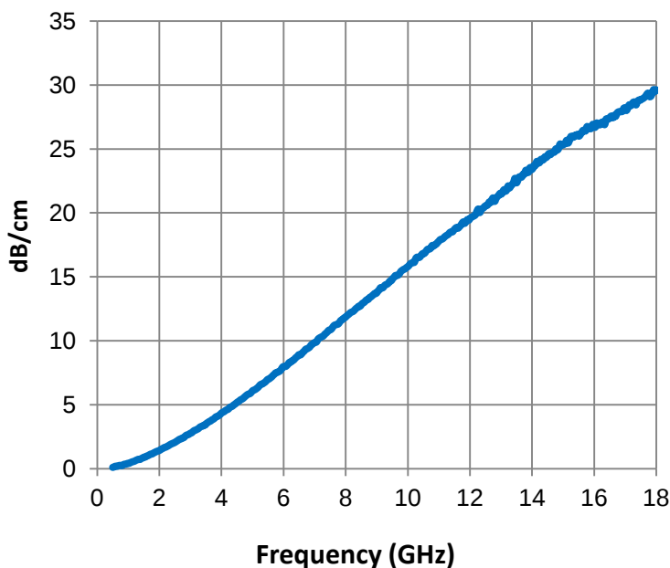
Attenuation
